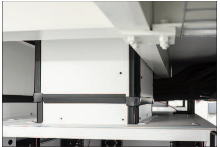
CPI 定制垂直排气管可隔离、重新输送和再循环热废气，以改善冷却低效问题。
